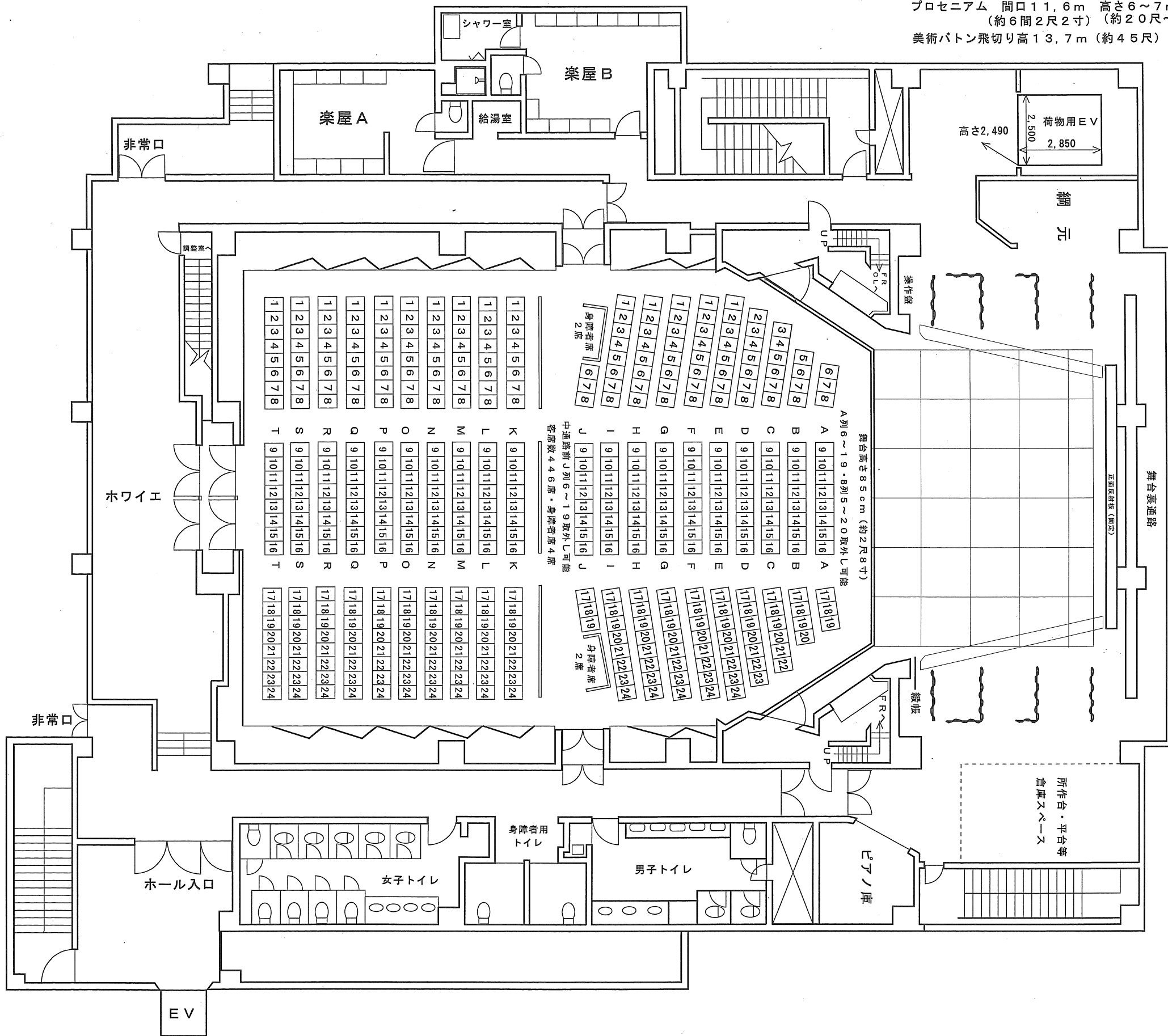
中川文化小劇場平面図 NO SCALE
